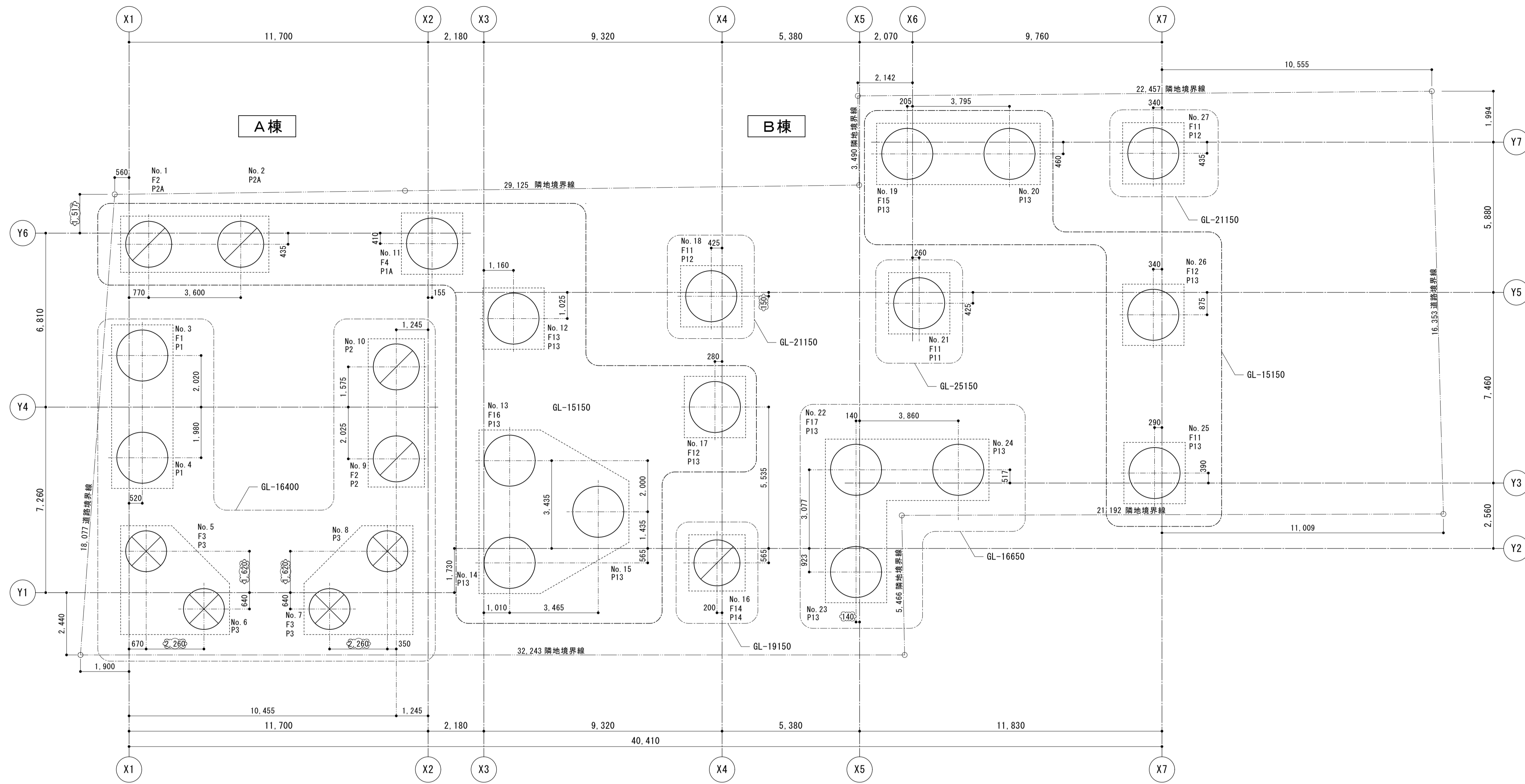
現場打ち杭の場合
