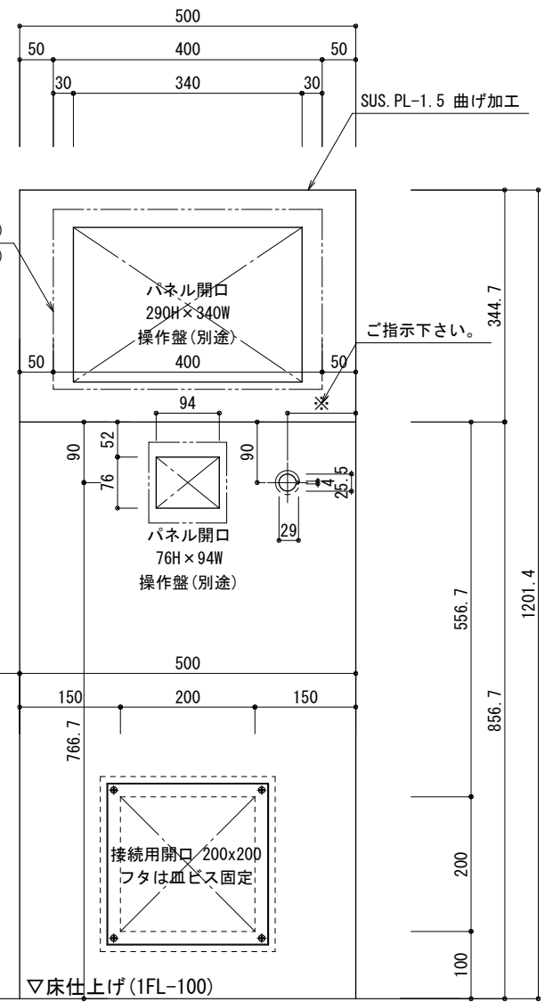
立面図(正面) S=1/5
