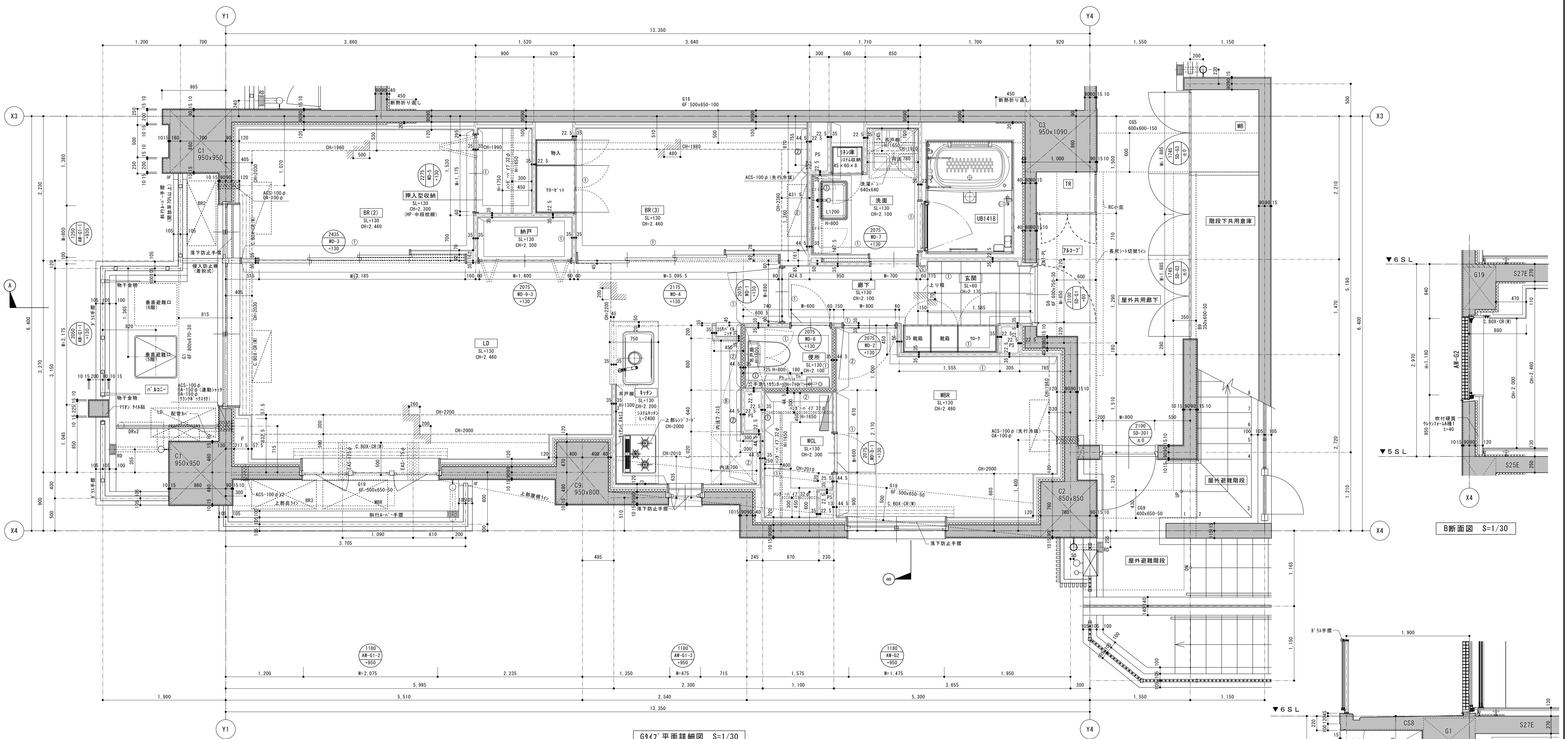
G17 平面詳細図 S=1/30
