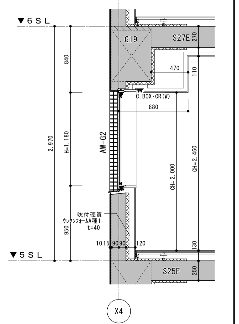
B断面図 S=1/30
