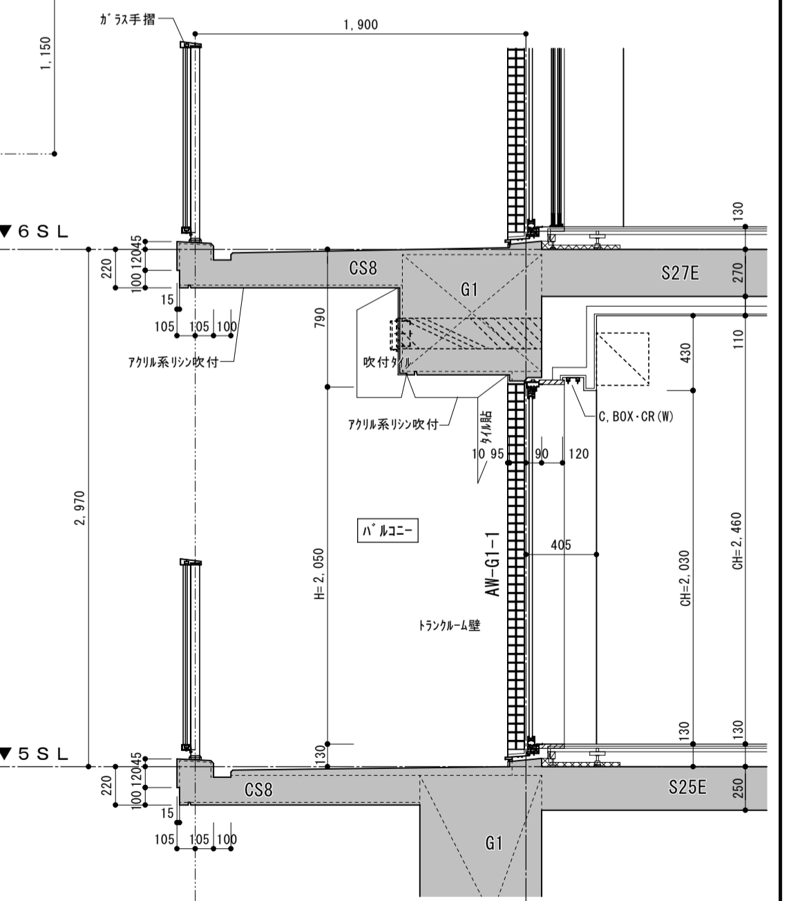
A断面図 S=1/30
